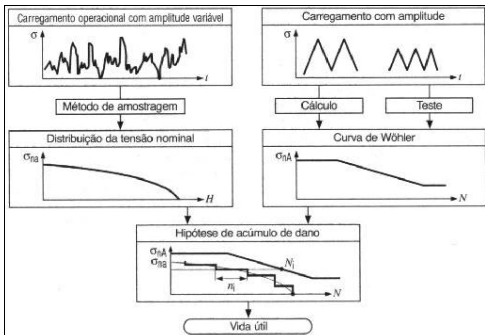
Figura 22: Procedimento para a análise da integridade operacional baseado no conceito de tensão nominal.
