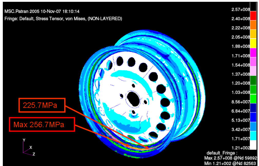
Figura 45: Carregamento a 0°
